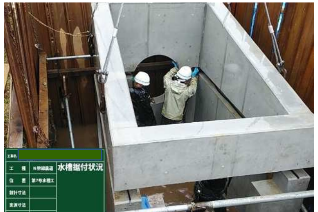
二分割水槽据付状況全景
