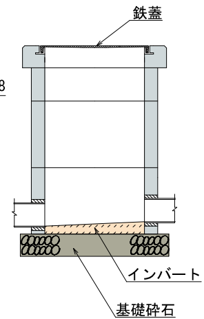
汚水柵施工例
