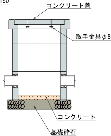
雨水柵施工例
