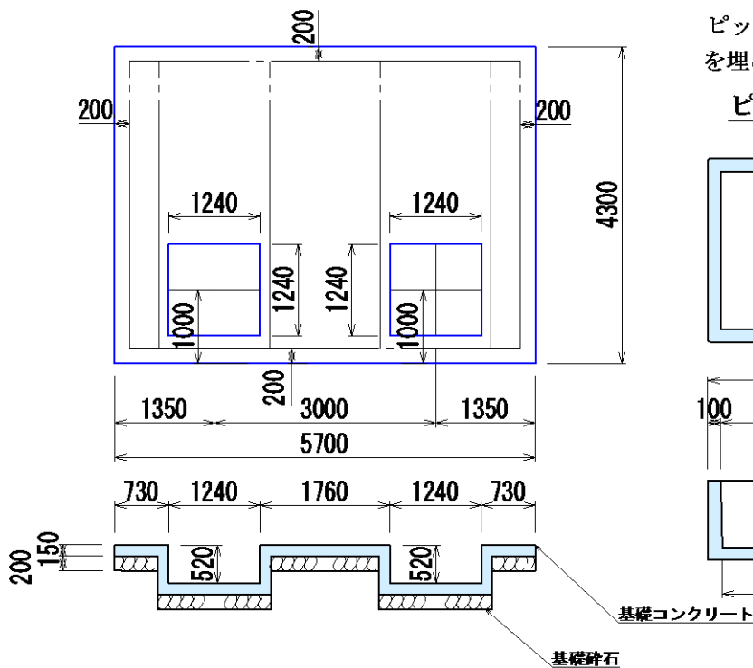
B型：標準基礎図
