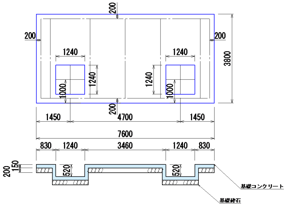
B型：標準基礎図
