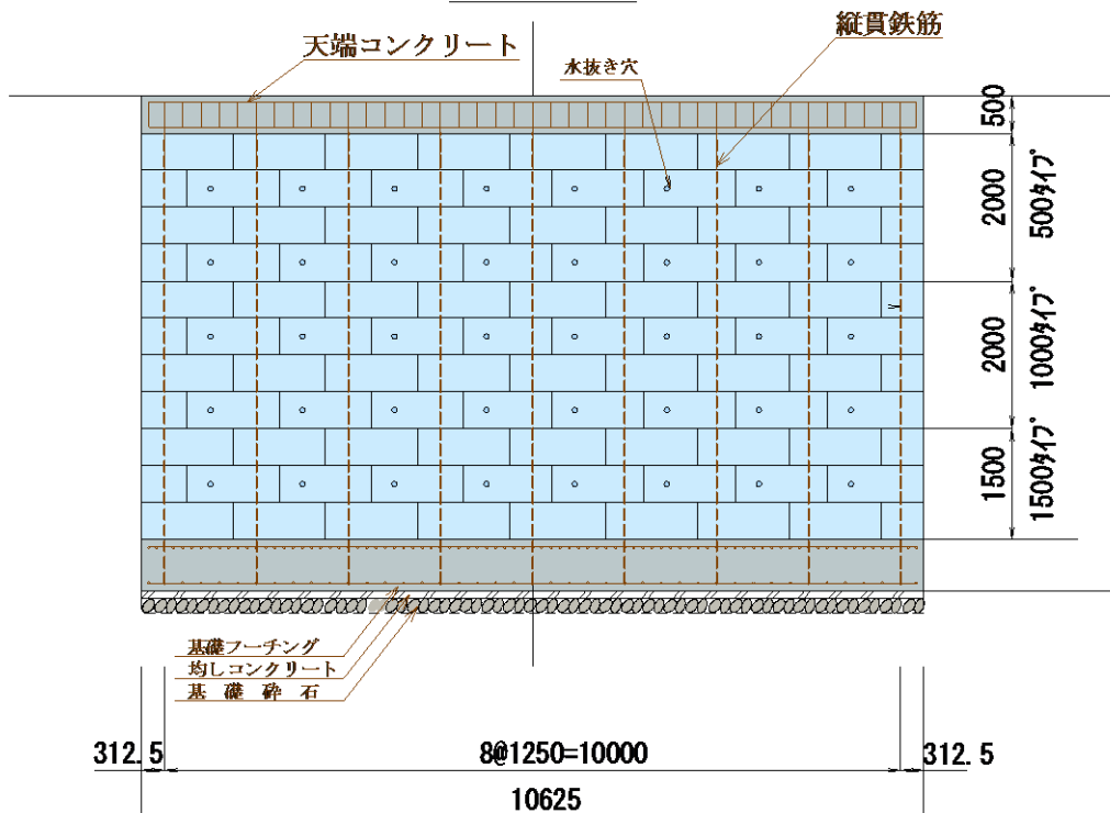
正面展開図
