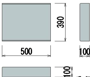
FC用コンクリート蓋
