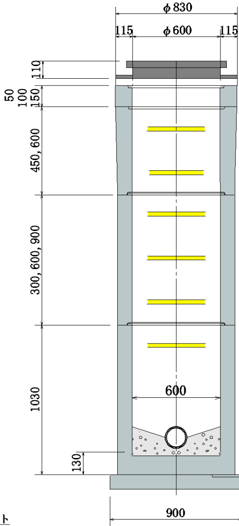
B-B断面図
