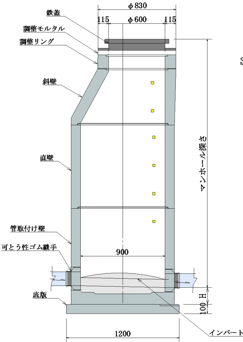
A-A断面図
