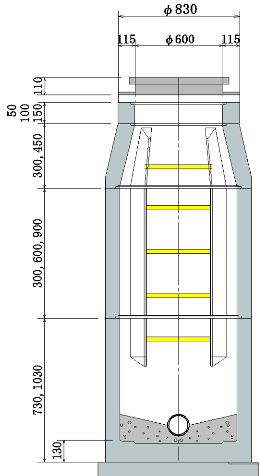
B-B断面図
