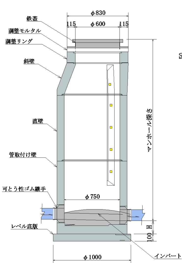
A-A断面図
