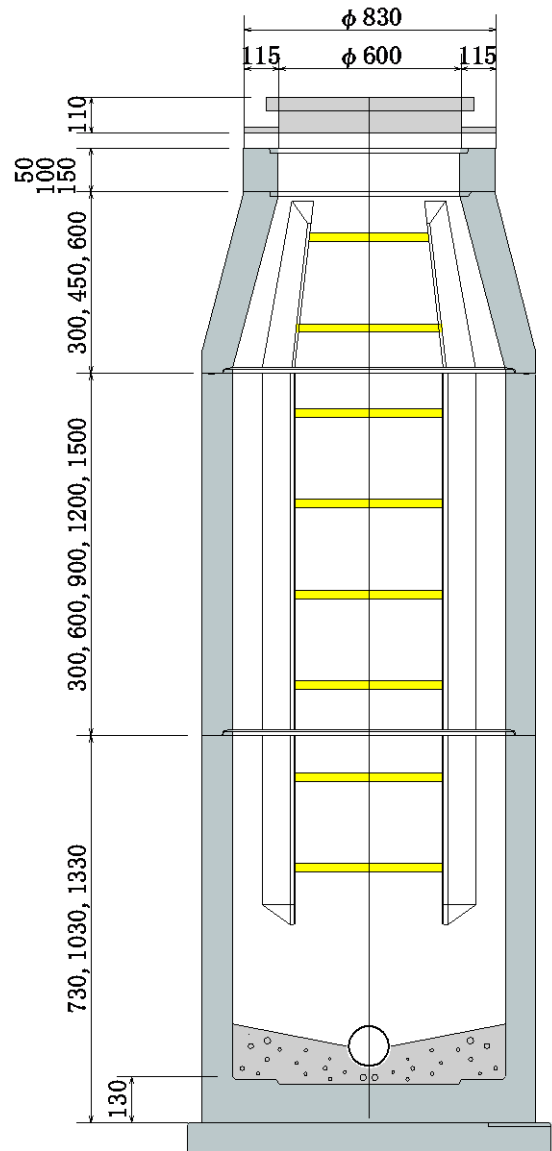
B-B断面図
