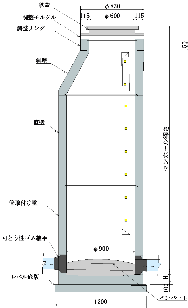
A-A断面図
