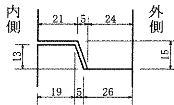
インロー部詳細図
